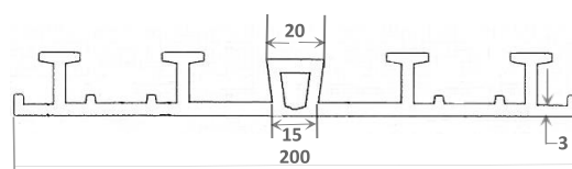
CL-Waterstop PV24200
